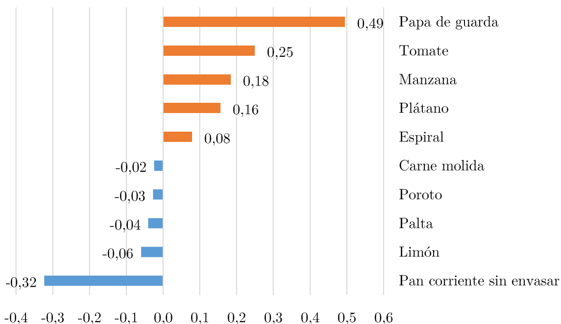
Figura 3 Productos con mayor incidencia positiva y negativa en la variación mensual de la CBA en agosto 2023
